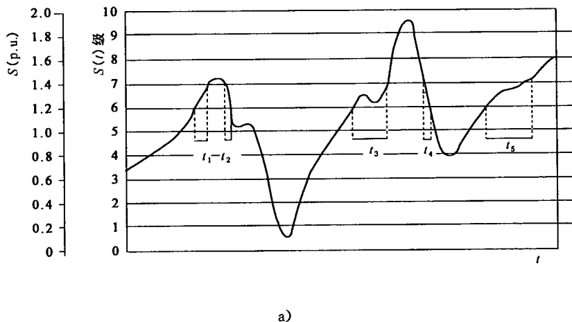
a) 图 A.2 由 S(t) 曲线作出的 CPF 曲线示例
